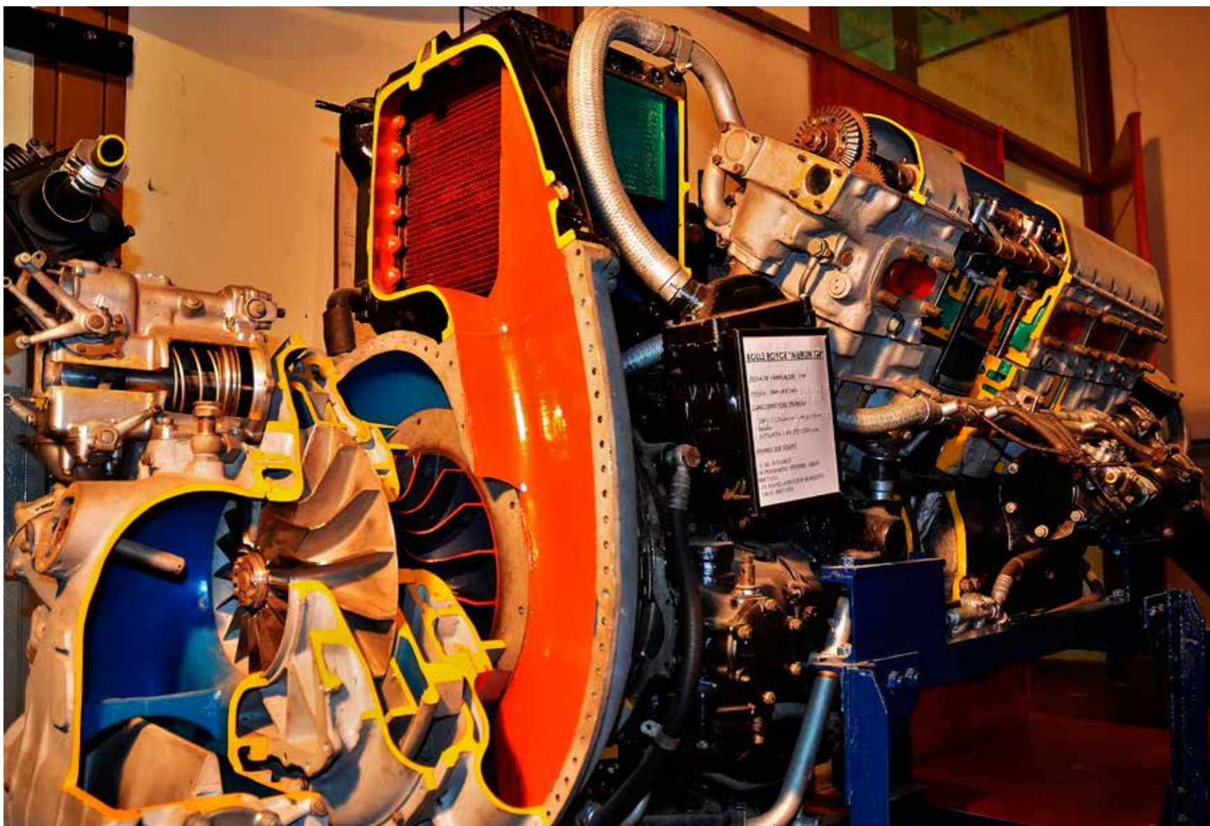
Motor Aeronáutico Rolls Royce Merlin 134.
